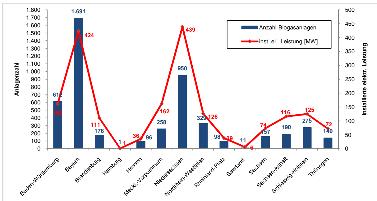
Anzahl Biogasanlagen und installierte el. Leistung [MW] nach Ländern (Stand: 12/2009)
